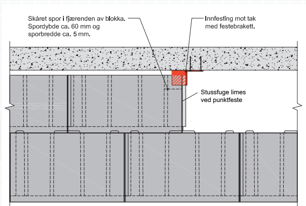
Figur A.2.10 Skjult innfesting til betongdekke med Leca Lettegg Toppforankring.
