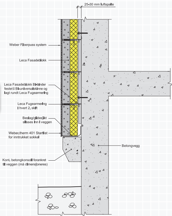
Figur A.10.4 Opplegg for Leca Fasadeblokk på betongkonsoll. Forblending mot eksisterende betongvegg.
