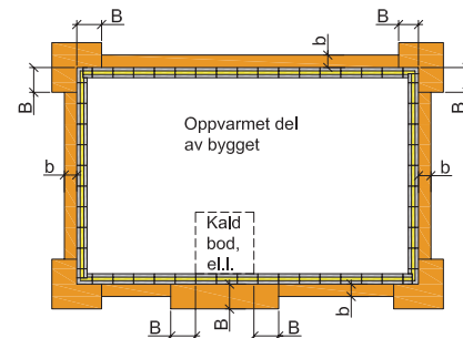
Figur D.8.1 Nødvendig markisolasjon med Leca Iso 10-20.
