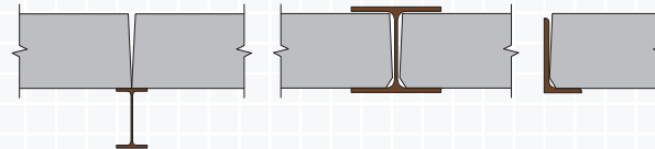
Figur C.2.10 Opplégg på stålbejelker. Elementene kan både legges inn i bejelken, og på toppflensen.
