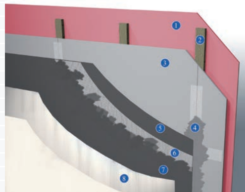
Figur B.9.1 Weber Luftet Kledning.
