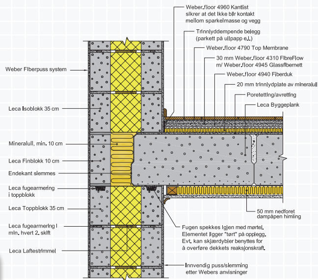
Figur C.2.3 Leca Lyddekte spenner parallelt med yttervegg i Leca Isoblokk 35 cm. For detaljer på lydøsning se kap C3 og C4. Tilfredsstill klasse C i NS 3475.
