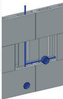
Figur A.2.19 Leca Lettvegg med innlagte trekkerør for skjult elektrisk anlegg.
