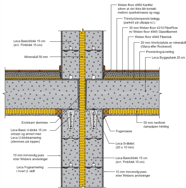
Figur A.3.10 Leca Lyddেকে opplagt på dobbeltvegg i Leca murverk.
