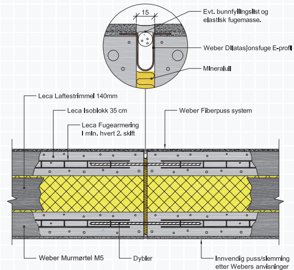
Figur A.9.1 Bevegesesfuge med skjærdybel.
