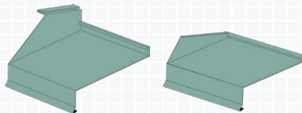
Figur A.11.2 I hver ende av sålbengkbeslaget lages en fals for tilpasning inn i mørtelfuge eller pussjikt. I bakkant lages oppbrett opp mot vinduets underside.
