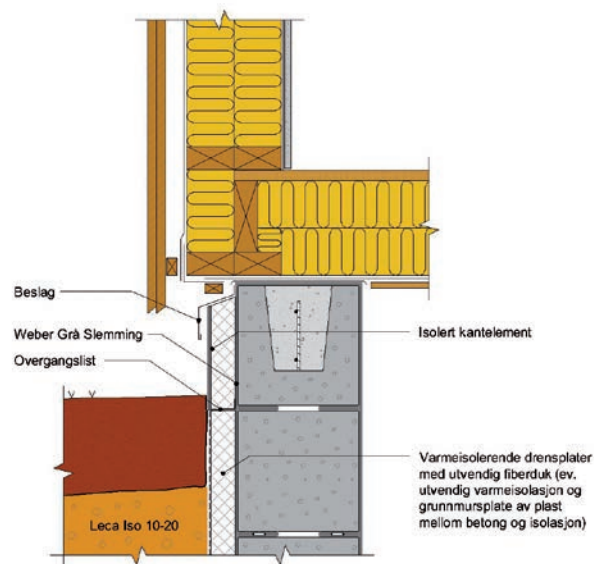
Figur B.5.6 Forslag til løsning for etterisolering av grunnmur i skrånende terreng (sokkel med økende høyde). Muren skal slemmes med weber Grå Slemming. Varmeisolerende dremsplater monteres iht leverandørens anvisning. Benytt egnet fiberpudd etter isolasjonsleverandørens anbefaling.
