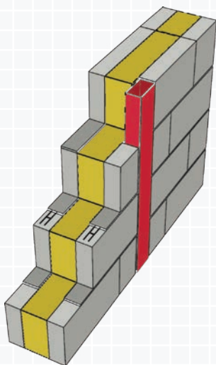
Figur A.9.4 Innmurt stålstender i indre vange på Leca Isoblokk. Pusses innvendig veggflate, bør pussen fiberarmeres min. 250 mm til hver side for stålsøylen i hele vegg høyden.
