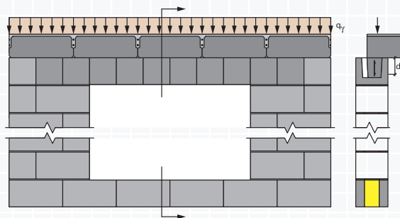
Figur A.5.14 Overdekning utført med ett armert og utstøpt U-blokkskift i murverk av Leca Isoblokk.
