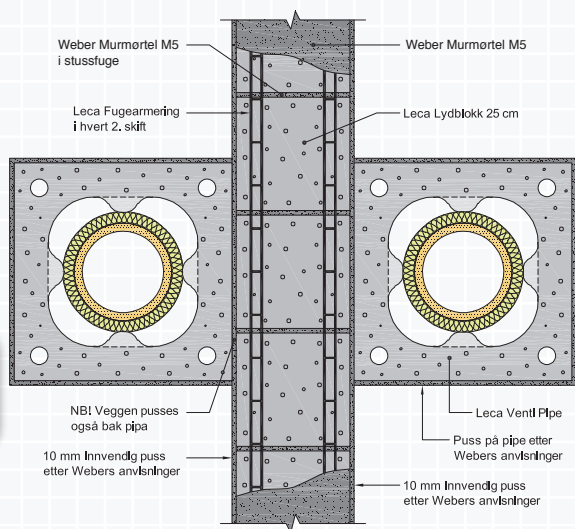
Figur A.8.6 Leca Venti Pipe mot lydskillevegg av Leca Lydblokk.
