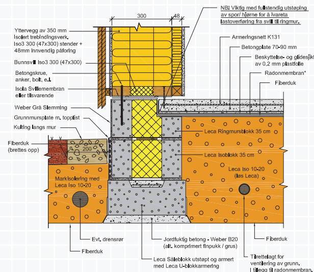
Figur A.6.1 Ringmur av Leca Ringmursblokk 35 cm med bunnsvill og stenderverk av Moelven Iso3 300 (47x300). Gulv på grunn med løs Leca og betongplate.
