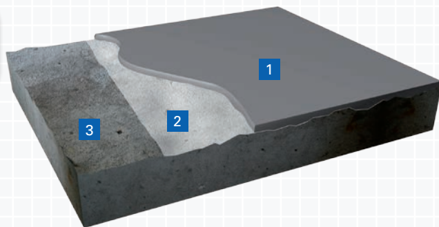
Figur C.6.1 Avretting på betong.
