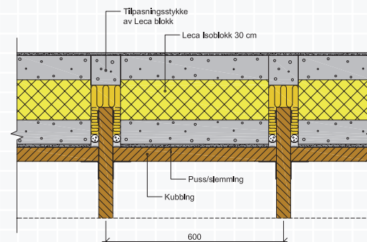
Snitt A-A (sett ovenfra)
