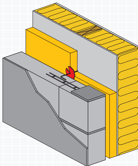
Figur A.10.3 Forblending med tilleggisolasjon (murplate), mot platekledning.
