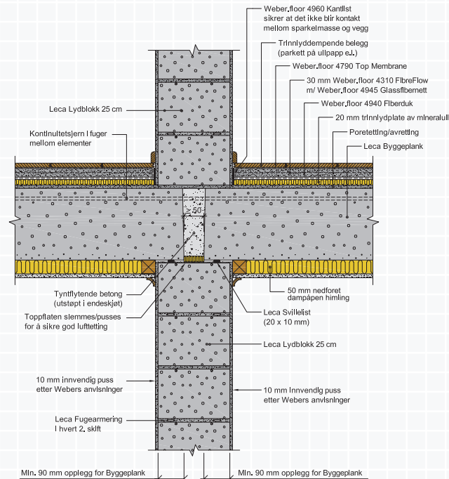
Figur A.8.3 Leca Lyddeke opplagt på lydskillevegg av Leca Lydblokk.
