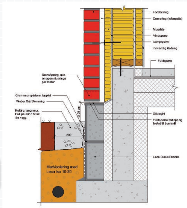
Figur B.5.7 Løsning for etterisolering av fasade og sokkel med bruk av Leca Blokk/Finblokk. Det benyttes weber Grå Slemming på sokkelen. Se ellers detaljer som beskrevet i standardløsningen i Figur B.5.2.
