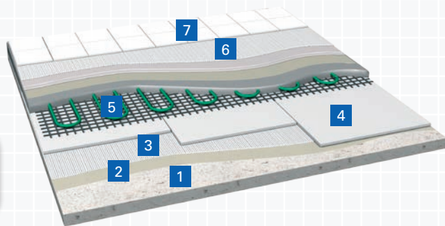
Figur E.5.1 Fliser på trinnlydsreduserende plate.
