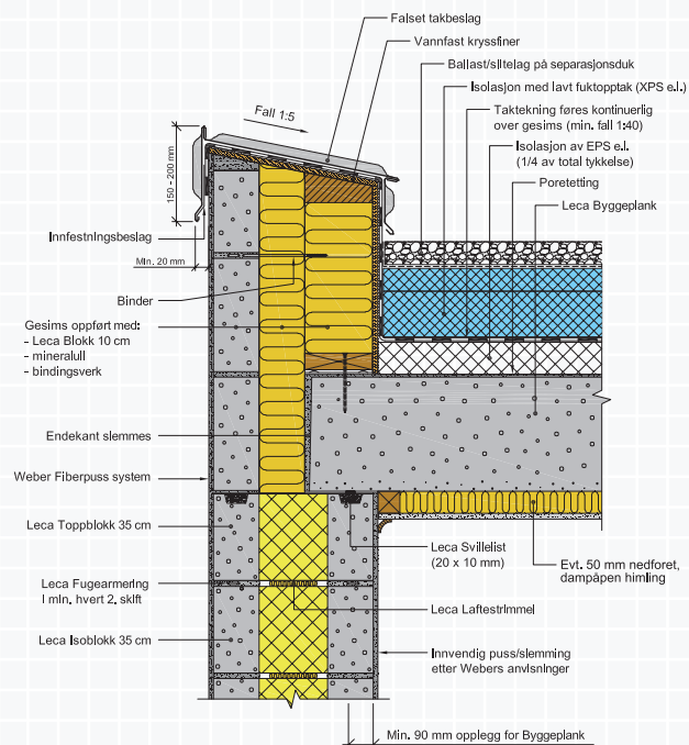
Figur C.2.15 Takavslutning med Leca Byggeplank. Duo løsning.
