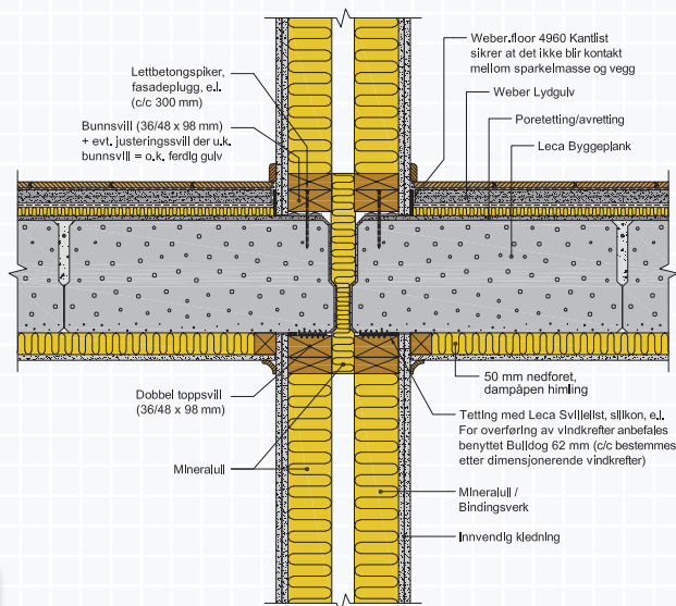
Figur C.2.9 Leca Lyddekke spenner parallelt med lydskillevegg i dobbelt 98 mm bindingsverk. Detalj for overføring av vindkrefter. For detaljer på lydløsning se kap C3 og C4. Tilfredsstiller klasse C i NS 8175.
