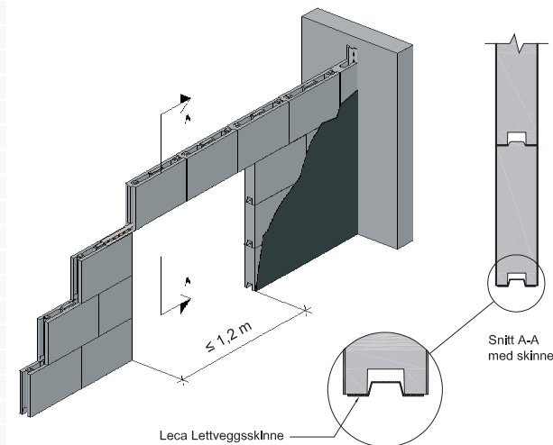
Figur A.2.11 Overdekning med understøttelse av Weber Letteggsskinne. Det anbefales å benytte lim i vertikalfugene.
