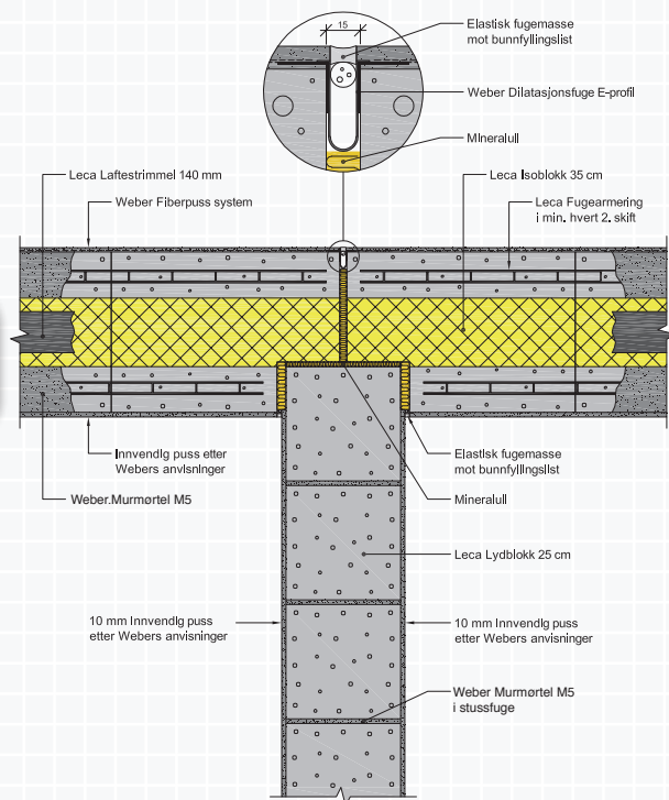
Figur A.8.4 Lydskillevegg av Leca Lydblokk mot yttervegg av Leca Isoblokk 35 cm. Løsningen anbefales kun over terreng pga. manglende tverravstivning mot jordtrykk.
