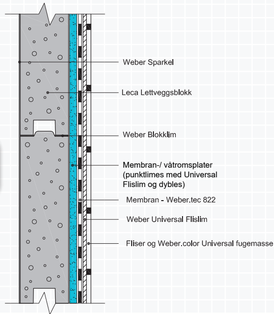
Figur A.2.24 Leca Lettvegg med membran/våtromsplater.
