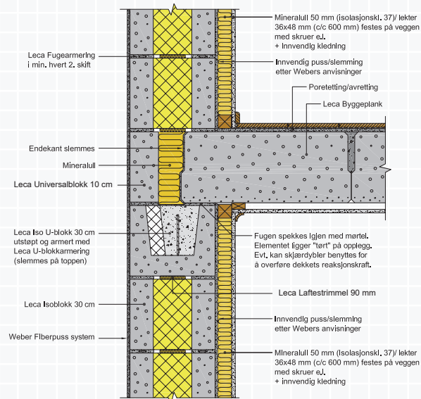
Figur A.5.8 Leca Byggeplank som spanner parallelt med yttervegg i Leca Isoblokk 30 cm.
