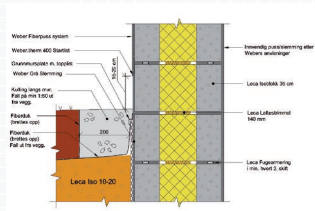
Figur B.5.2 Standardløsning for Leca grunnmur. Dreneringsplate med topplister avsluttes under bakkenivå. Bak dreneringsplate og opp til minimum 25 cm over bakkenivå benyttes weber Grå Slemming. Fiberpussystemet starter med Startlist. Se Figur B.5.3 for detalj i overgang slemmemørtel/Fiberpuss.
