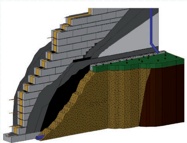
Figur B.5.1 Prinsipp av grunnmur. 5 forutsetninger for beskyttelse av grunnmur og fasade er tegnet inn. (Ikke i målestokk).
