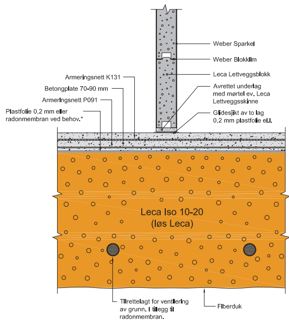
Figur D.2.5 Innvendig ikke-bærende Leca Lettvegg.
