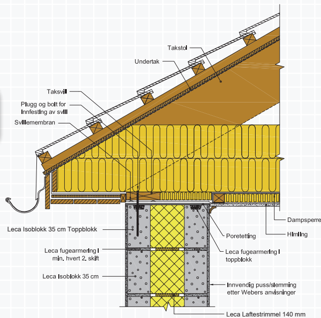
Figur A.4.10 Opplegg for tretak på yttervegg i Leca Isoblokk 35 cm.
