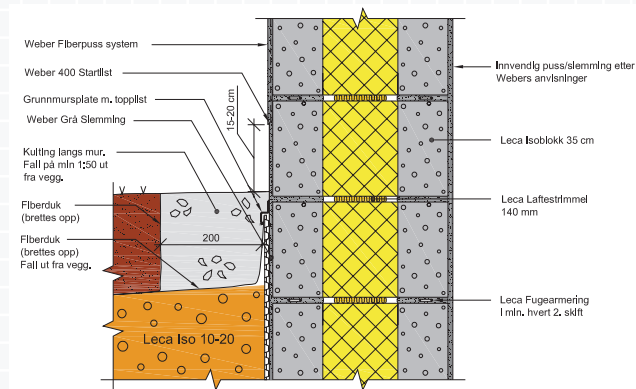
Figur B.5.4 Prinsippskisse for montering av beslag ned mot fast dekke/ belegningsstein. Beslaget skal i toppen freses på skrå oppover i puss/underlag og overlappe grunnmursplaten.
