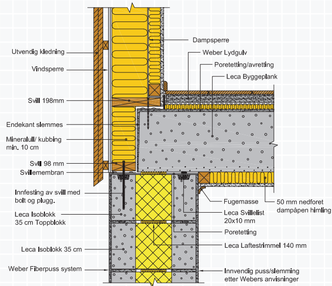
Figur A.4.5 Leca Lyddeke på grunnmur av Leca Isoblokk 35 cm.
