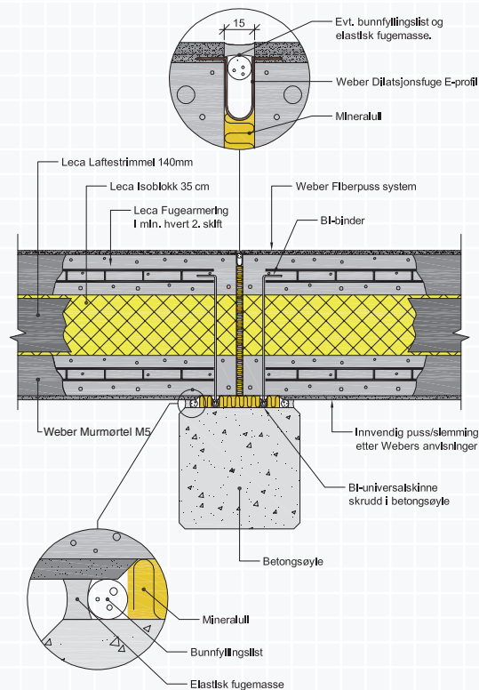
Figur A.9.9 Forankring av Leca Isoblokkvegg til avstivende betongsøyle med BI-forankringssystem. Bevegelsesfuger avsettes ved behov.
