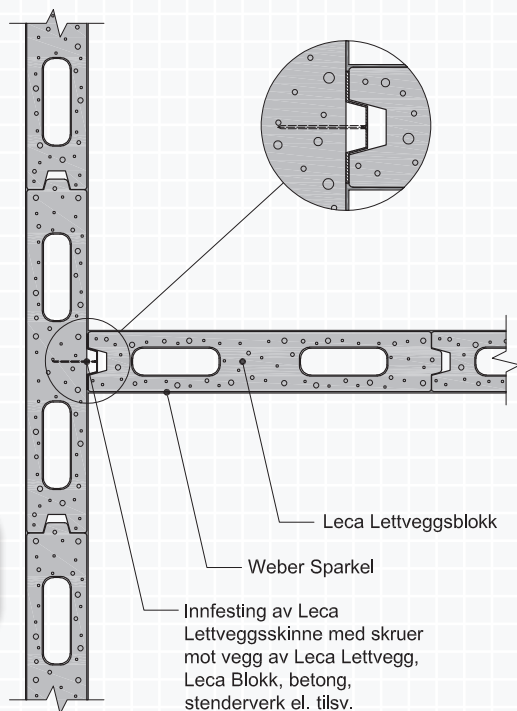
Fig. A.2.6 Horisontalsnitt som viser innfesting av Leca Lettvegg mot en Leca Lettvegg ved bruk av Leca Lettvegsskinne og skruer/spiker. Skinnen blir dekket helt av sporet i Leca Lettveggsblokk.
