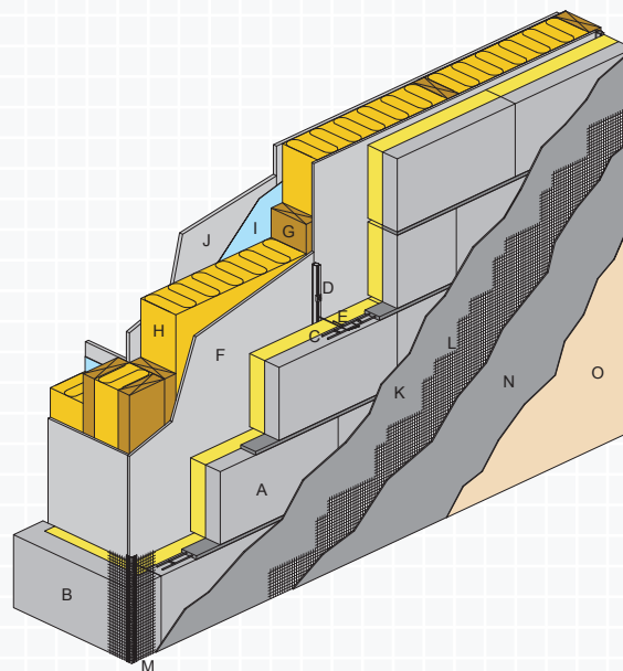
Figur A.10.1 Forblending med pusset Leca Fasadeblokk. Bakenforliggende vegg i isolert trebindingsverk.
