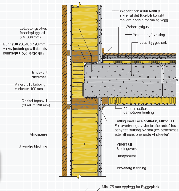
Figur C.2.5 Leca Lyddekke spenner parallelt med yttervegg i 198 mm bindingsverk. Detalj for overføring av vindkrefter. For detaljer på lydøsning se kap C3 og C4. Tilfredsstiller klasse C i NS 8175.
