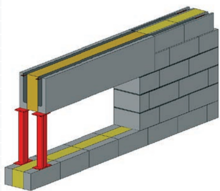
Figur A.4.18 Stålsøyler med fordelingsplater. Søylene og fordelingen av punktlaster må dimensjoneres særskilt.
