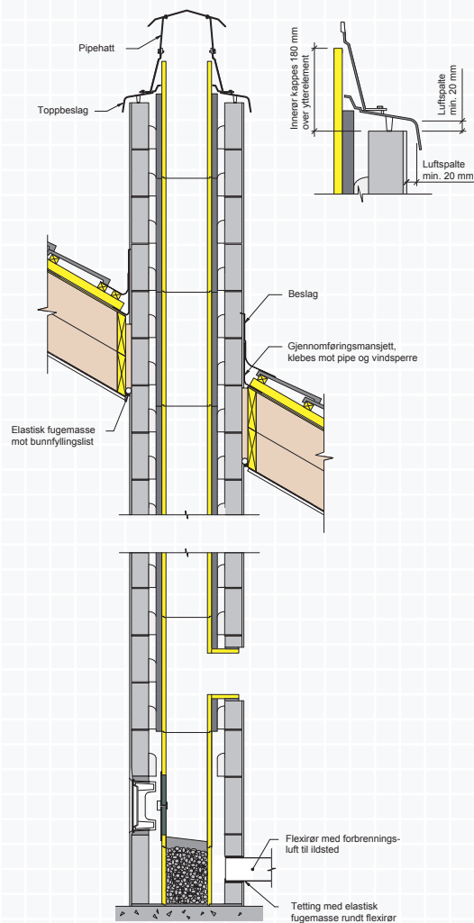
Figur F.3.6 Lufttetting ved taggjennomføring. Detalj av luftspalte ved toppbeslag. NB! Prinsippfigur, plassering av tilluftsstuss og sotlukeåpning tilpasses i hvert enkelt tilfelle.
