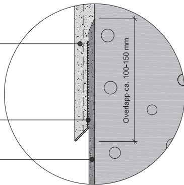
Figur B.5.3 Detaljskisse av overgang mellom weber Grå Slemming og Weber Fiberpuss systemet. Overlappen er ca 15 cm med weber 400 Startlist som festes mekanisk med egnet rustfri stift. Startlisten fungerer som pusslire, pen avslutning og beskyttelse av Fiberpussen.
