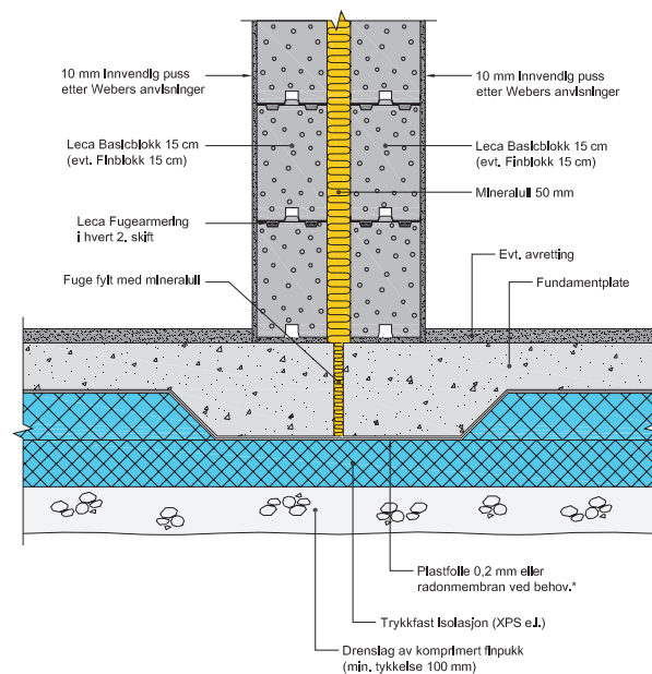
Figur A.3.9 Dobbeltvegg i Leca mellom to bruksenheter skilt med gjennomgående fuge fylt med mineralull.
