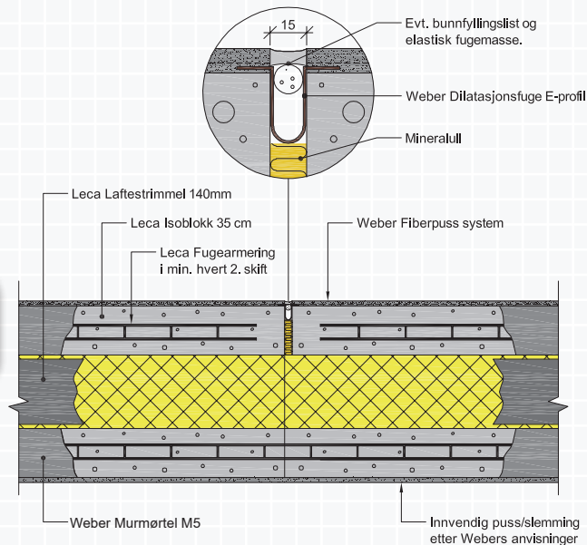
Figur A.9.2 Bevegesfuge i ytre vange i Leca Isoblokkvegg.
