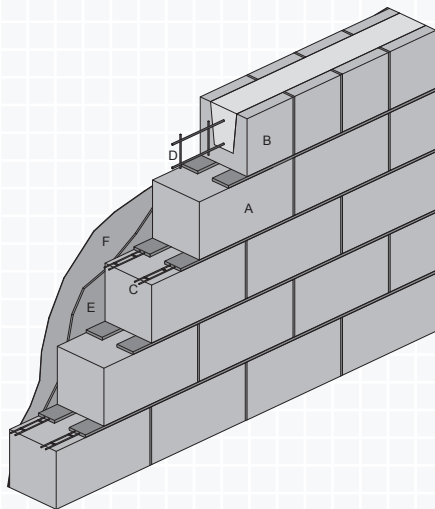
Figur A.7.2 Innervegg av Leca Finblokk 20 cm med delte ligge- og stussfuger. Pusset på én side og fuget/spekkmurt på den andre siden.
