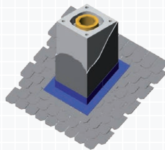
Figur F.9.1 Pipebeslag for flatt takbelegg.
