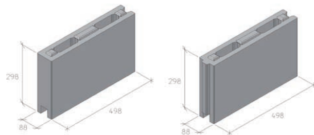
Figur A.2.1 Leca Lettvegsblokk 88 mm og Leca Lettvegg Hjørneblokk 88 mm.
