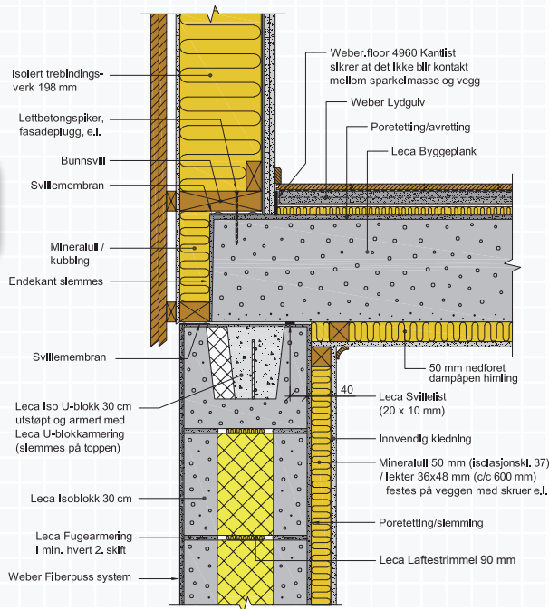
Figur A.5.5 Leca Lyddekte på grunnmur av tilleggisolert Leca Isoblokk 30 cm.
