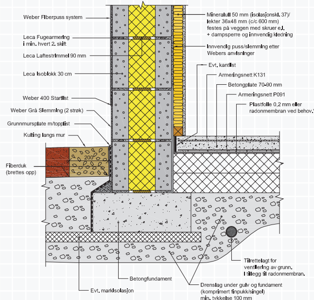
Figur A.5.4 Veggopplegg for Leca Isoblokk 30 cm på støpt betongsåle.
