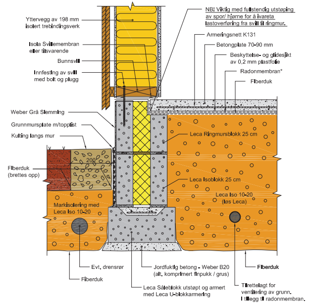
Figur D.2.4 Leca Ringmur 25 cm.
