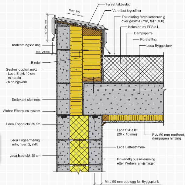
Figur C.2.14 Takavslutning med Leca Byggeplank. Løsning med rettventd, kompakt tak.
