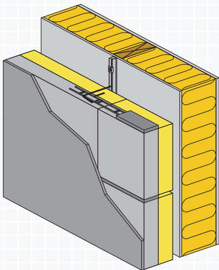
Figur A.10.2 Forblending med Leca Fasadeblokk, mot platekledning.
