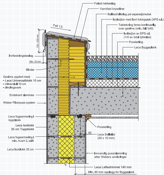
Figur A.4.11 Takavslutning med Leca Byggeplank.
