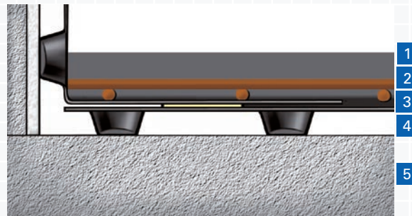
Figur C.6.8 Fuktsperre med luftspaltende belegg.
