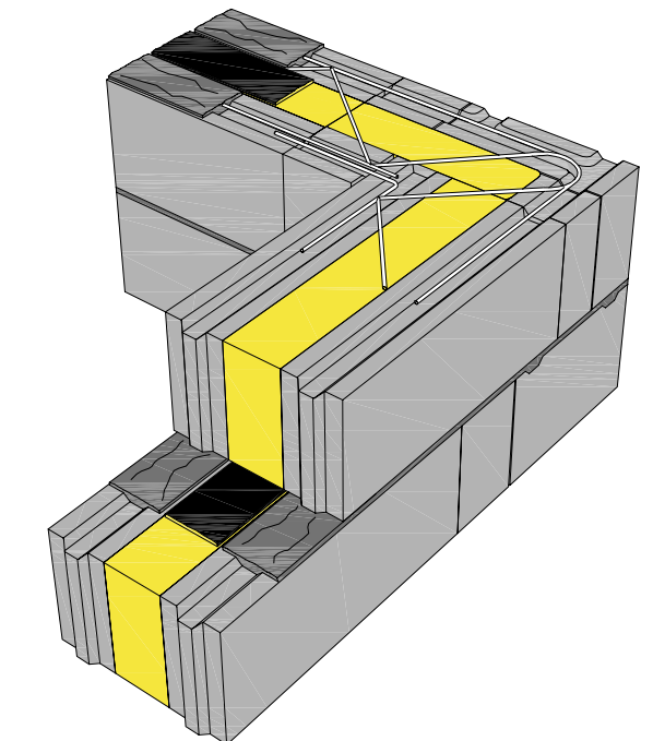
Figur 4.21 Leca Sikksakk-armering rundt hjørne
