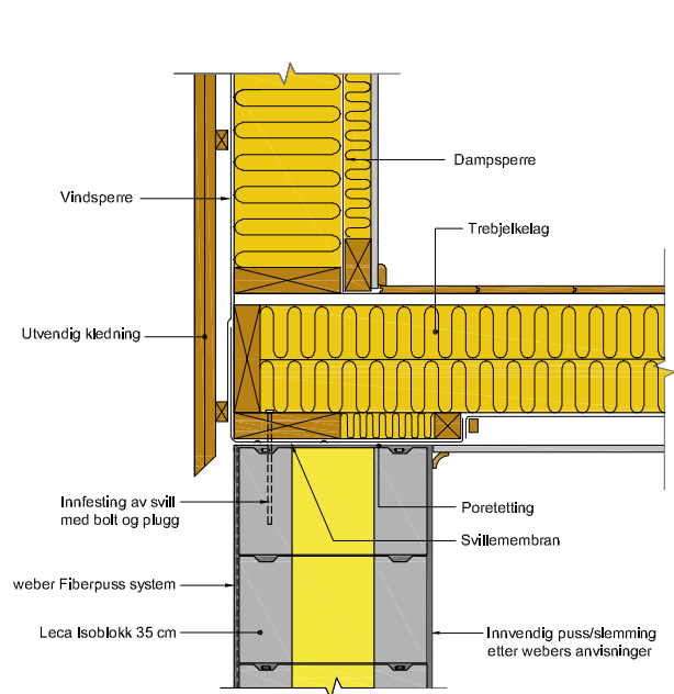
Figur 4.26 Opplegg for trebjelkelag på Isoblokk
