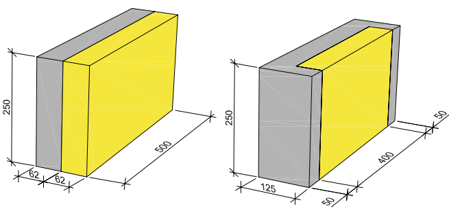
Figur 9.1 Leca Fasadeblokk – Blokkdimensjoner
