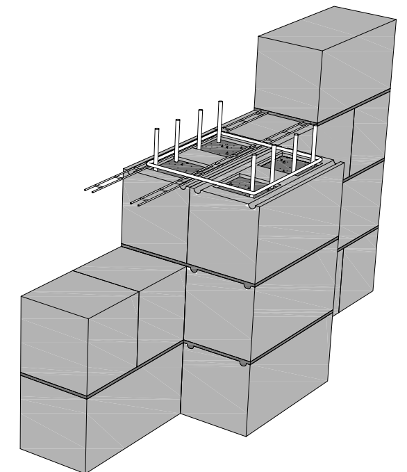
Figur 4.12 Pilaster av Leca Konstruksjonsblokk
