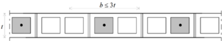
Fig. 7.7 Medvirkende trykksonebredde
