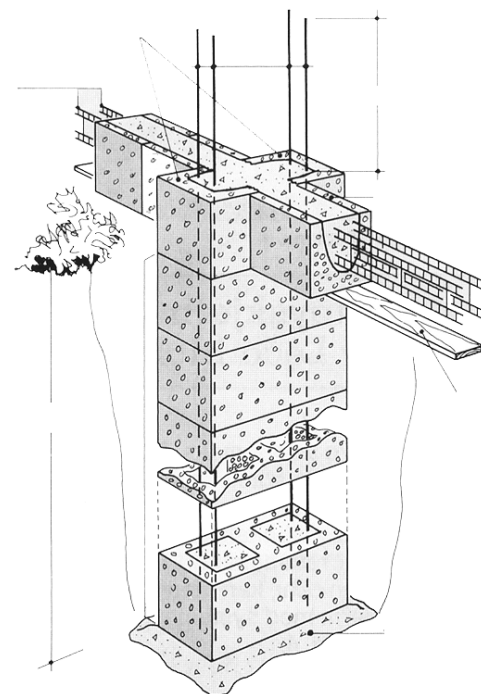
Figur 5.17 Fundament for murt skjerm med gjennomgående U-blokkskift
