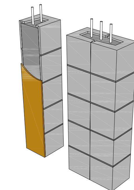
Figur 4.36 Søyler murt av Leca U-blokk på høykant
