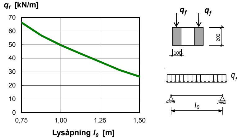
Diagram 7.72 Bæreevne for Leca Isobjelke komplett 20 cm
