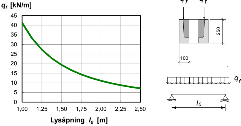
Diagram 7.71 Bæreevne for Leca Overdekningsbjelke 25 cm
