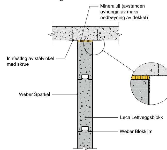
Figur 10.4a Innfesting til betongdekke med stålvinkler på hver side av veggen.
