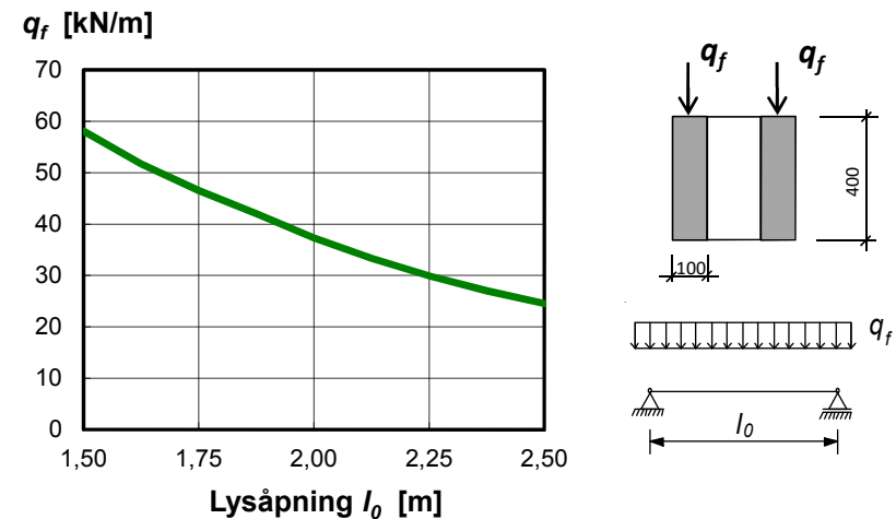
Diagram 7.73 Bæreevne for Leca Isobjelke komplett 40 cm
