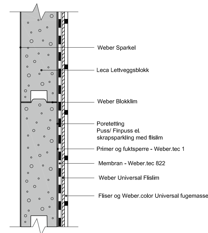
Figur 10.10a Leca Lettvegg med Weber Våtromssystem.
