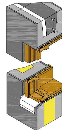
Figur 4.37 Vindu i yttervegg av Leca
