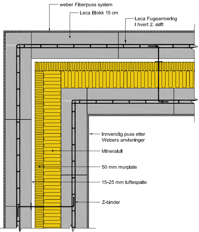
Figur 8.4 Skallmurvegg av Leca Blokk 15 cm. Plantegning
