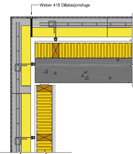
Figur 9.7 Forankring ved vertikal bevegelsesfuge i hjørne
