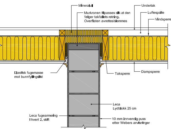
Figur 5.10 Veggavslutning mot tak
