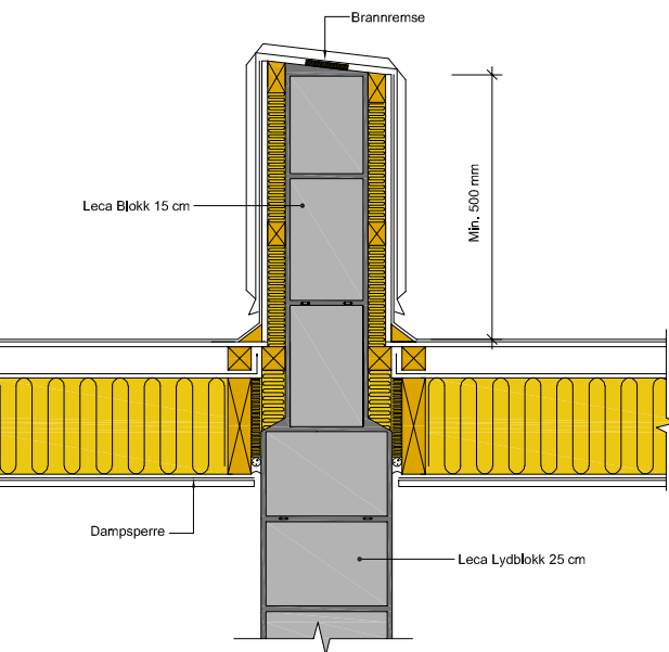
Figur 5.11 Lydskillevegg/brannvegg (REI 240) føres min. 500 mm over tak
