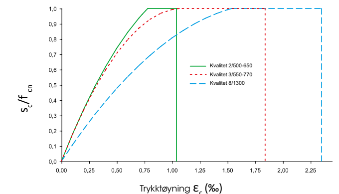
Figur 3.5 Karakteristisk arbeidsdiagram for Leca murverk med Leca Universalblokk ved vertikal trykkpåkjenning. Det antas at Leca LSX har tilsvarende verdier ved samme fasthet.
