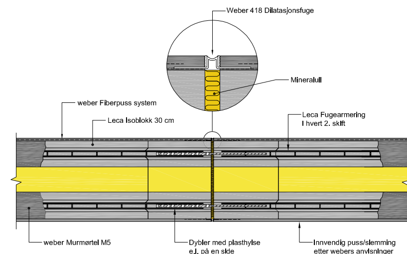
Figur 4.22 Bevegelsesfuge i Leca vegg
