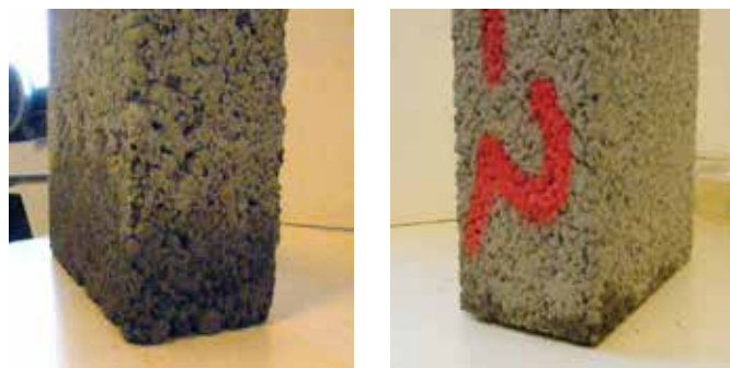
Figur 3.7 Vannoppsug test for Leca blokker av ulik type. Til venstre tradisjonell Leca blokk. Til høyre LSX blokk som viser klart redusert kapillær sugesevne.
