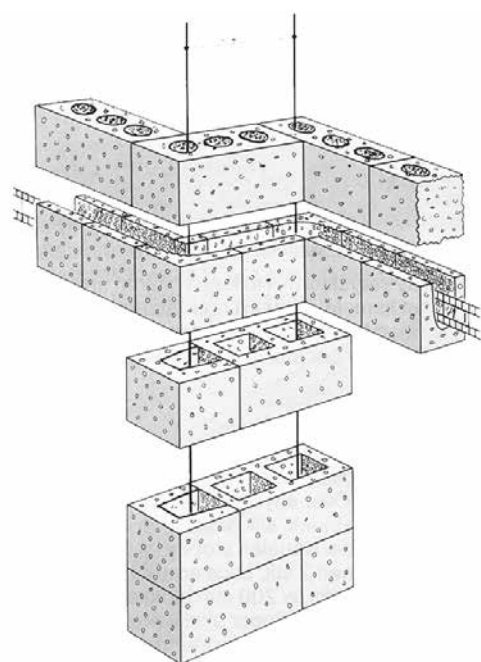
Figur 5.16 Murt vinkelskjem
