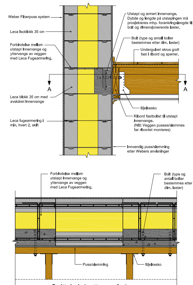
Figur 4.27 Skjult ribordløsning for trebjelkelag på Isoblokk
