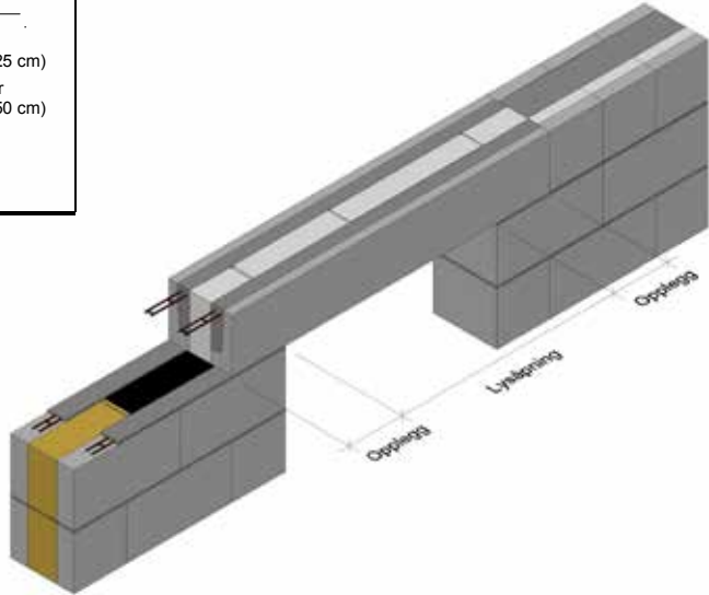
Leca Overdekningsbjelke
