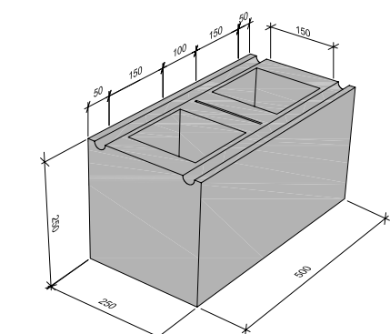
Figur 4.31 Leca Konstruksjonsblokk
