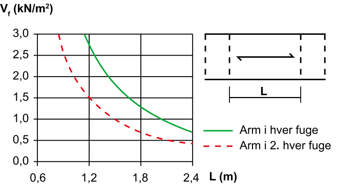
Figur 9.5 Maksimal avstand L (m) mellom forankringsskinner avhengig av belastning og armering (Leca Fugearmering) med dimensjonerende moment M f = v f * L² / 10
