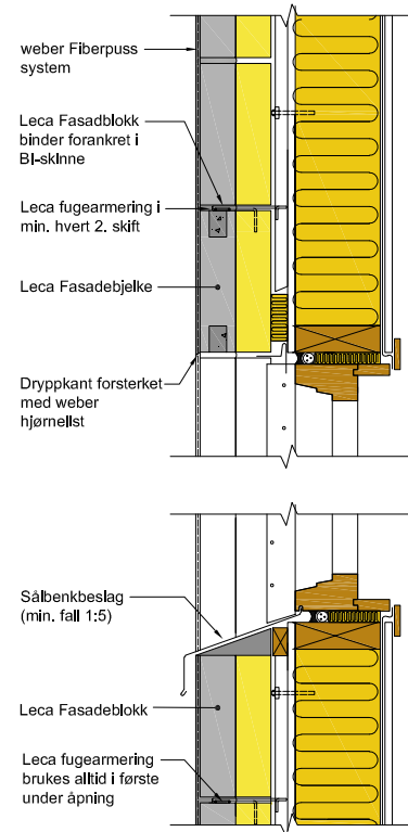
Figur 9.17 Vindusinnsetting i bakvegg av isolert bindingsverk – vertikalsnitt
