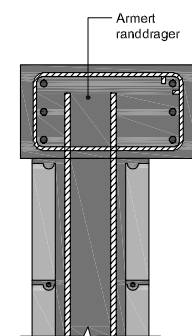
Figur 4.33b Vegg av Leca Konstruksjonsblokk. Toppavslutning med randdrager.
