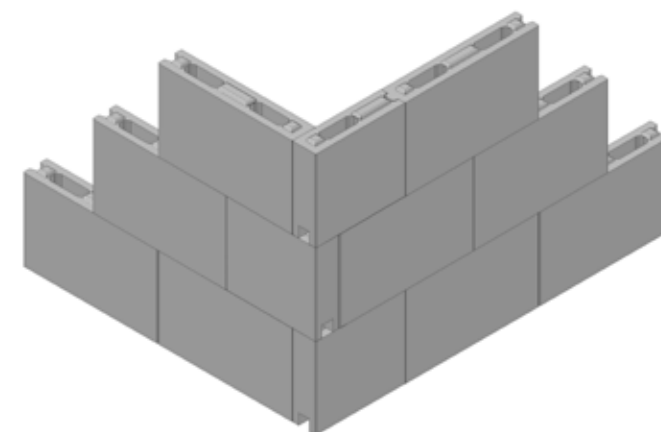
Figur 10.6c Hjørneløsning med 1/2 blokks forband.
