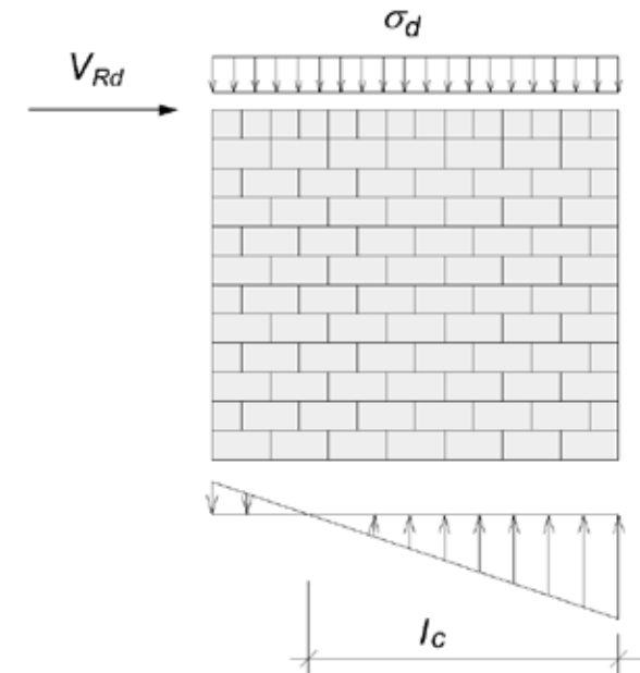
Figur 7.20 Stabiliserende veggskive i Leca murverk
