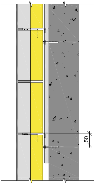
Figur 9.6 Plassering av BI-skinne og bindere i forhold til skifthøyden
