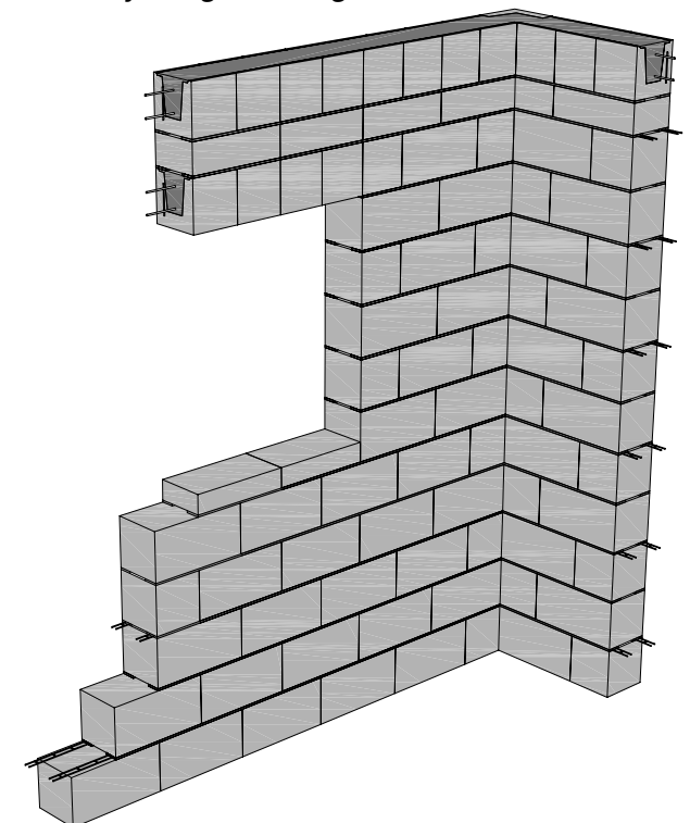
Figur 4.13 Armering av Leca murverk
