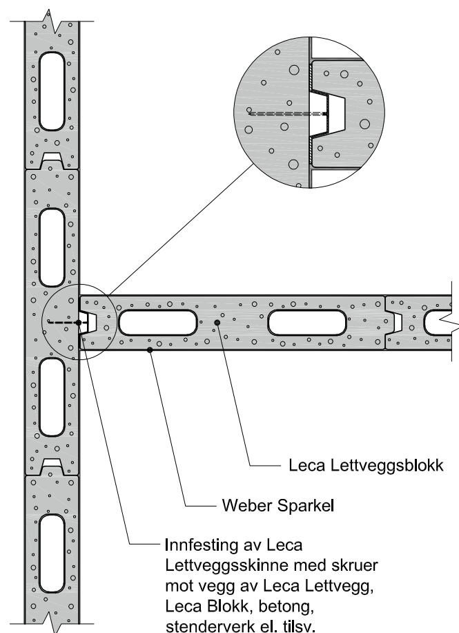
Fig. 10.3b Horisontalsnitt som viser innfesting av Leca Lettvegg mot en Leca Lettvegg ved bruk av Leca Lettveggsskinne og skruer/spiker. Skinnen blir dekket helt av sporet i Leca Lettveggblokk.
