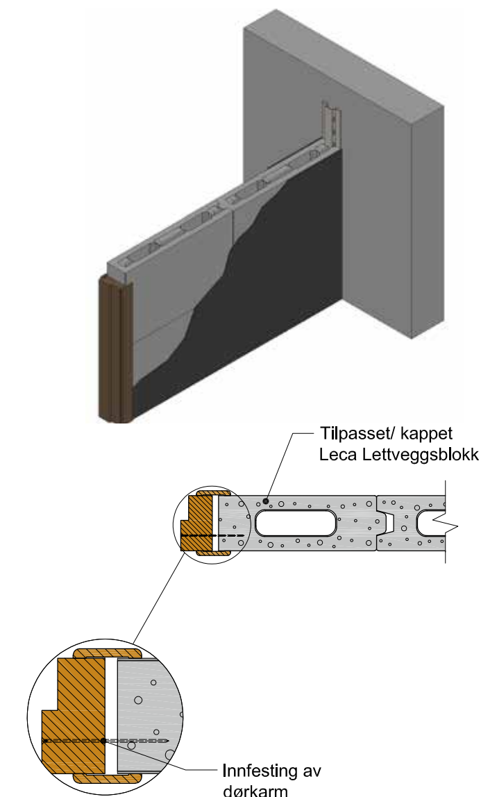
Figur 10.5d Innsetting av dør.
