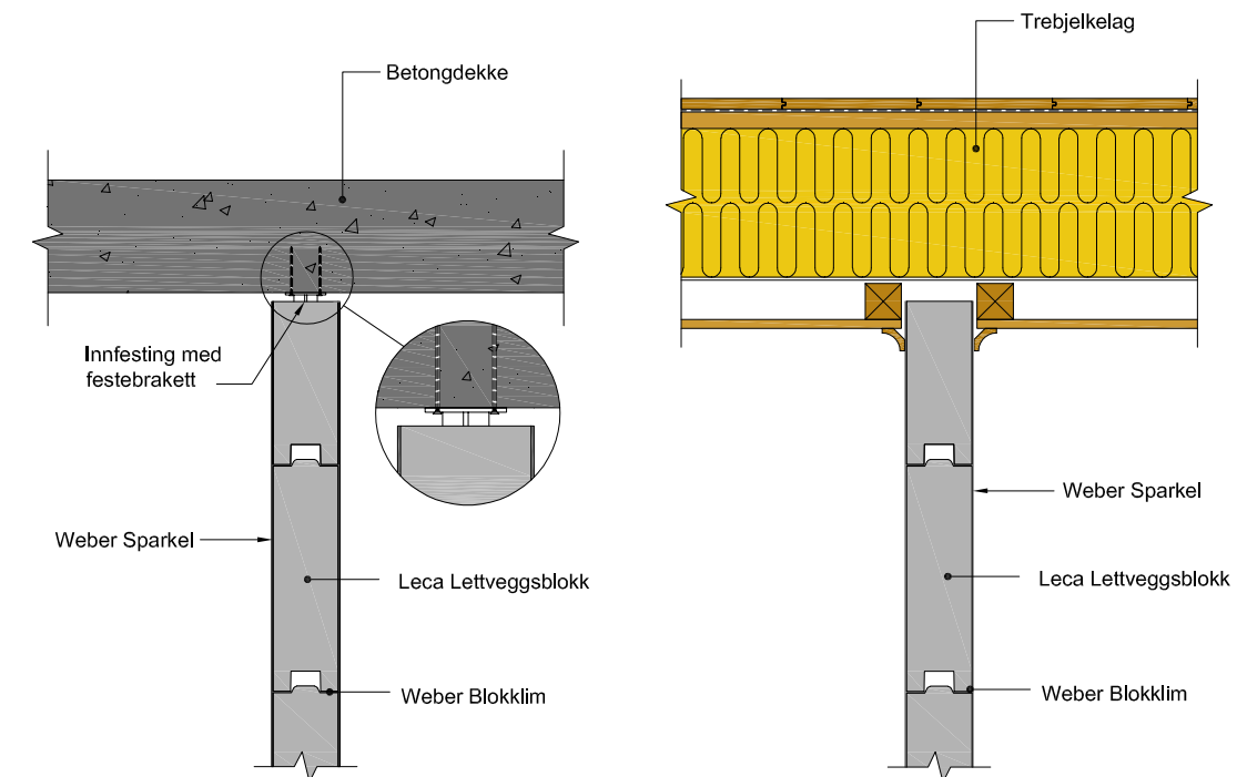
Figur 8.8 Innvendig bærevegg av Leca Finblokk 20 cm. Vertikalt snitt
