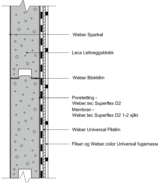
Figur 10.10b Leca Lettvegg med sementbasert membran fra Weber.
