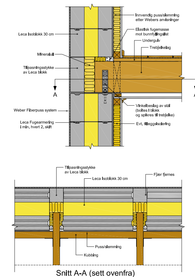
Figur 4.28b Opplegg av trebjelkelag på Isoblokk. Vekslet inn i murverk.
