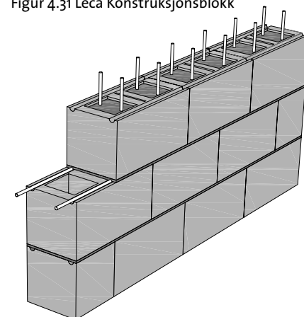
Figur 4.32 Murverk av Leca Konstruksjonsblokk. Armert og utstøpt
