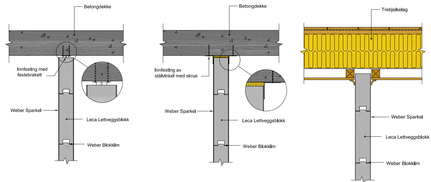
Figur 4.30 Veggavslutning mot betongdrager/dekke
