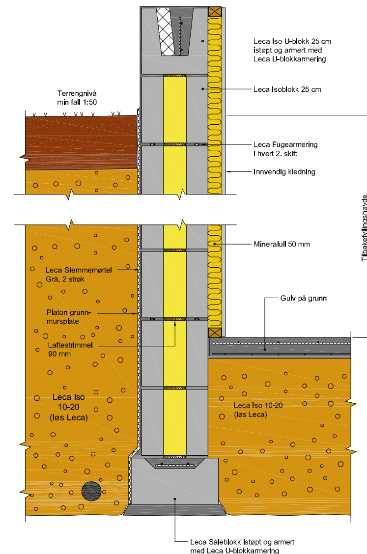
Figur 8.3 Sandwichvegg av Leca Isoblokk 25 cm under terreng, tilleggisolert 50 mm. Vertikalt snitt
