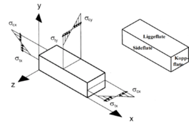
Fig. 7.1 Definisjon av mursteinsflater, akseretninger og normalspenninger i murverk
