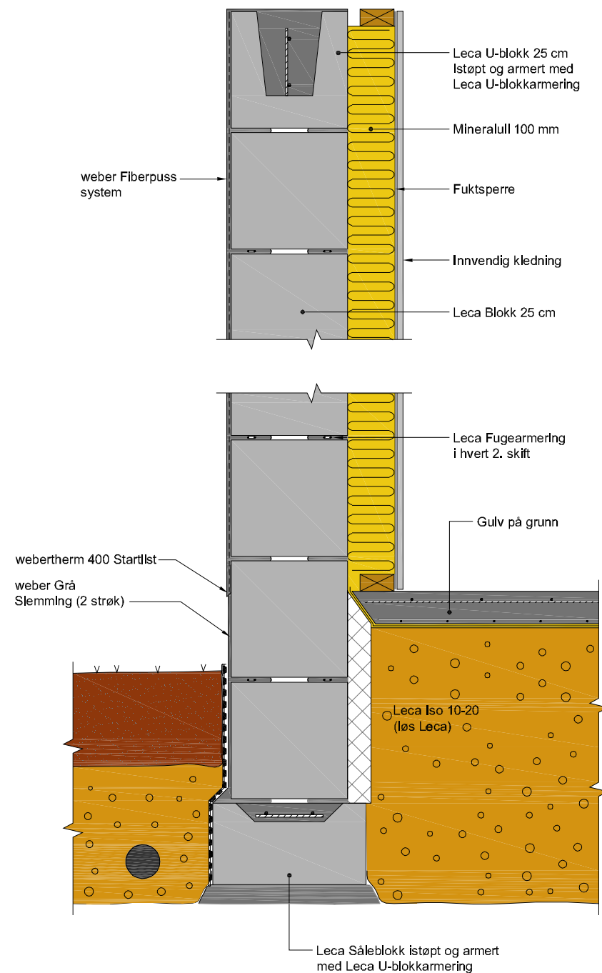
Figur 8.2 Massiv yttervegg av Leca Blokk 25 cm, tilleggisolert 100 mm. Vertikalt snitt. NB! Løsningen anbefales kun over terreng.
