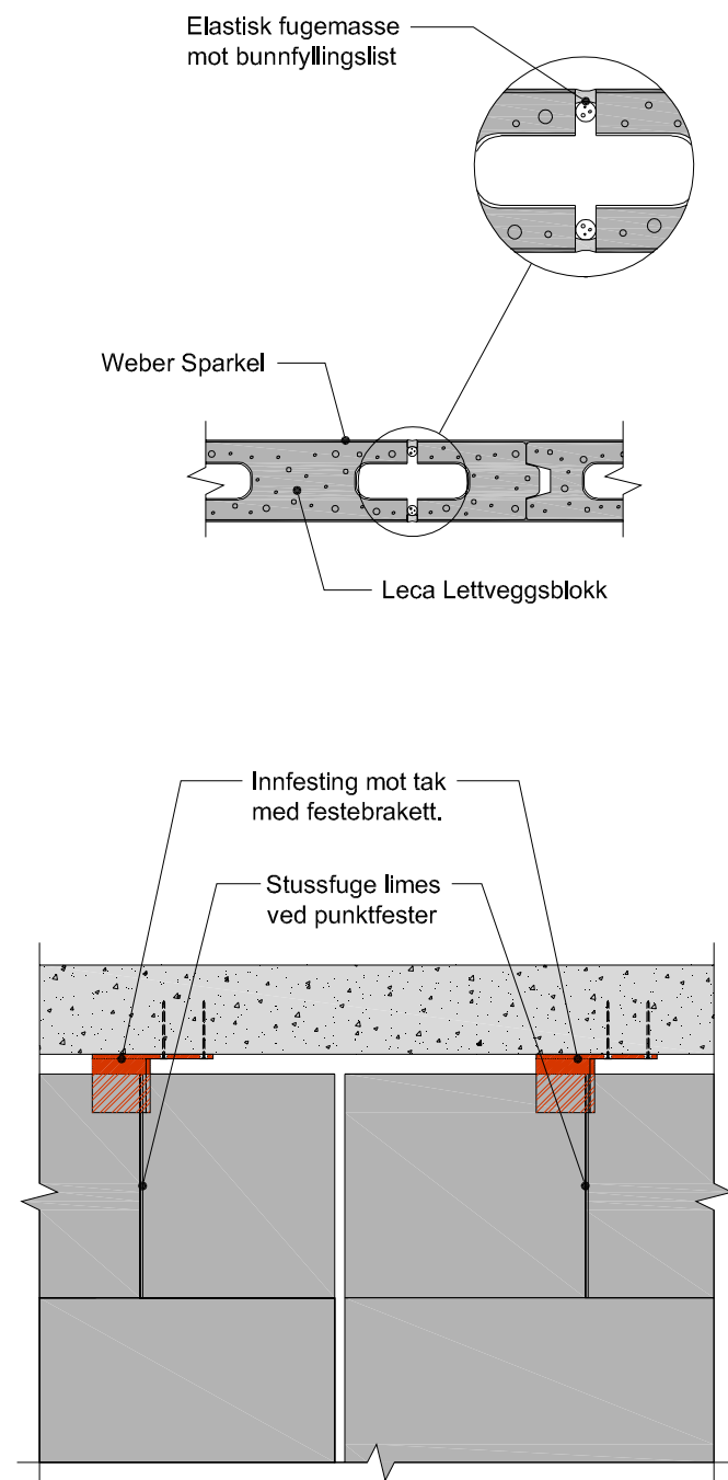
Figur 10.7 Bevegelsesfuger.
