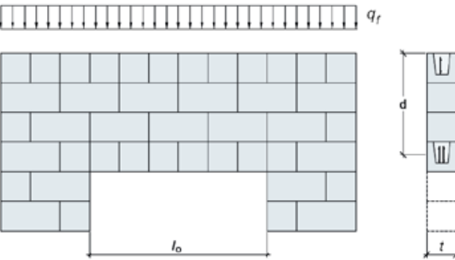
Figur 7.19 Murt overdekning
