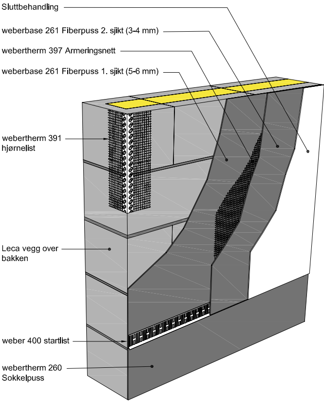
Figur 4.44 Weber Fiberpussystem
