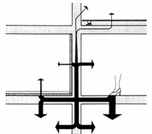
Figur 5.2 Trinnlydoverføring
