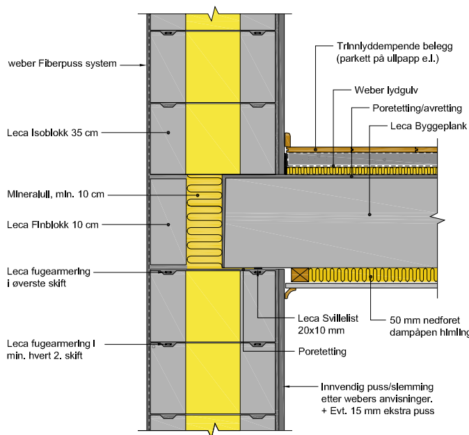
Figur 5.7 Overgang mellom Leca Lyddekke og yttervegg av Leca Isoblokk 35 cm
