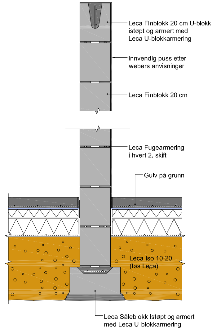
Figur 8.8 Innvendig bærevegg av Leca Finblokk 20 cm. Vertikalt snitt
