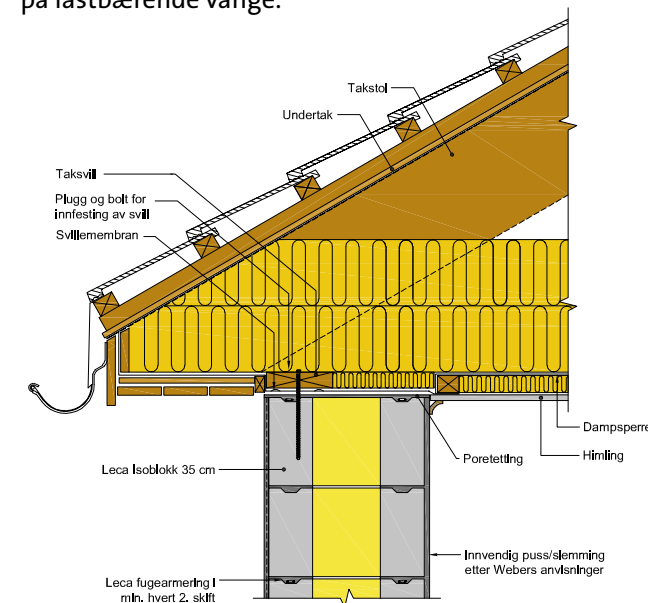
Figur 4.29 Opplegg for tretak på Isoblokk
