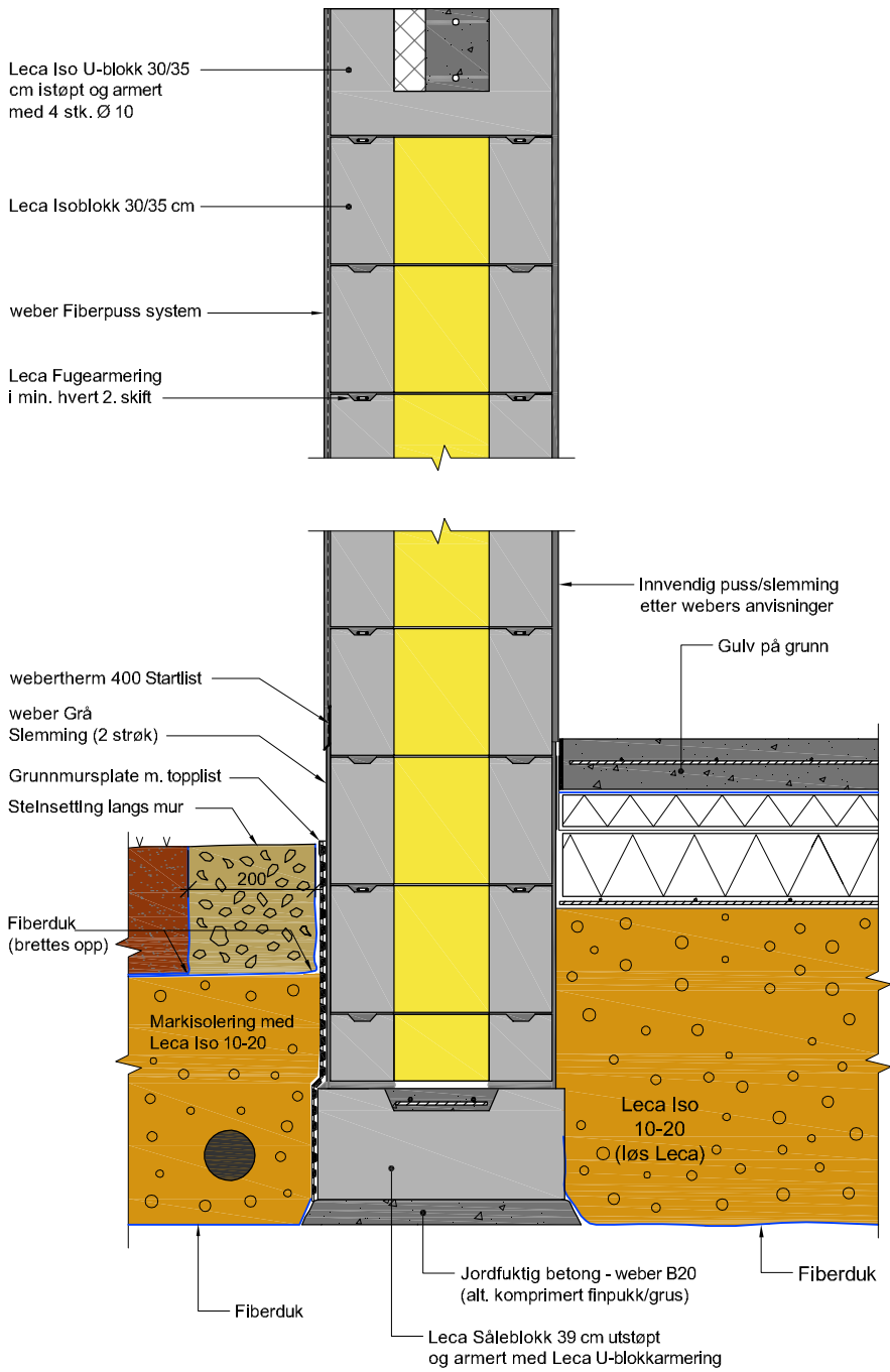
Figur 8.1 Sandwichvegg av Leca Isoblokk 35 cm. Vertikalt snitt
