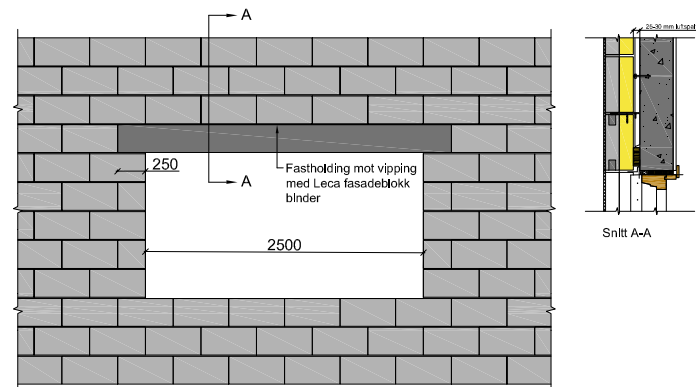
Figur 9.10 Leca Fasadebjelke
