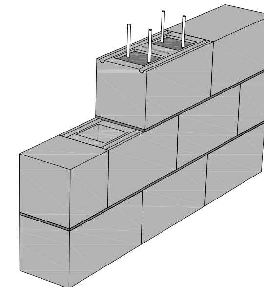
Figur 4.11 Innmurt Leca Konstruksjonsblokk
