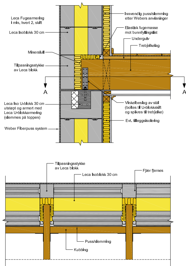
Figur 4.28a Opplegg av trebjelkelag på Isoblokk. Vekslet inn i murverk med U-blokk
