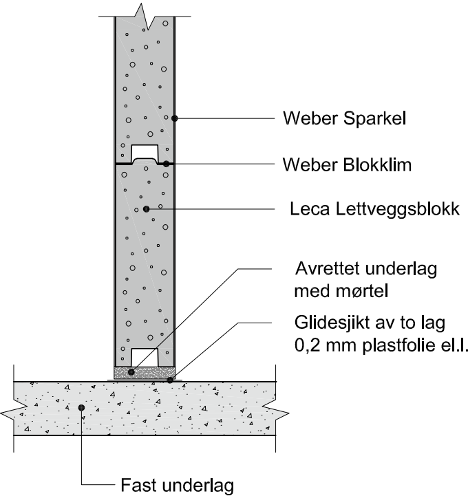
Figur 10.2a Leca Lettvegg på avrettet underlag/fundament.
