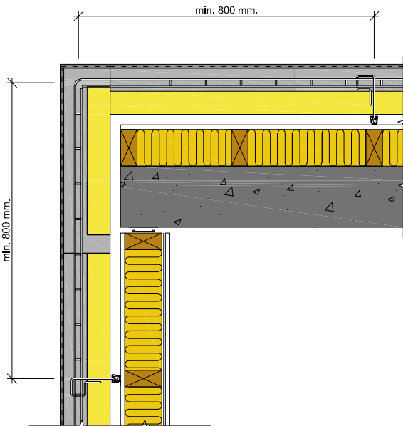
Figur 9.8 Forankring ved ommurt hjørne
