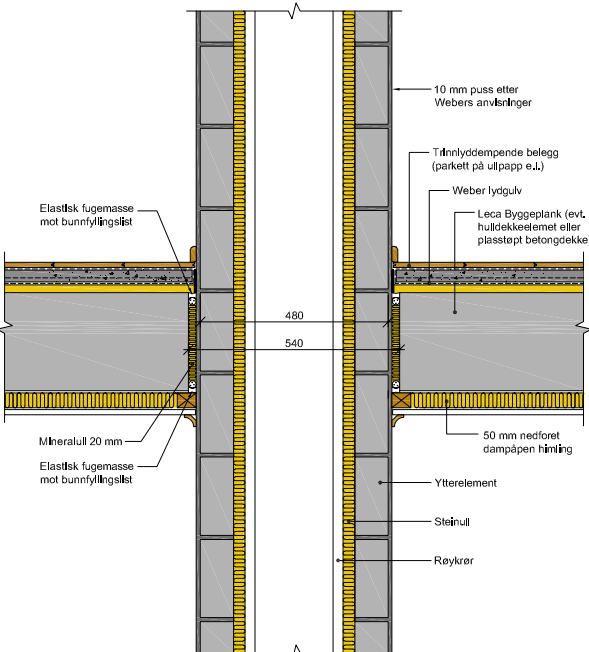
Figur 5.13 Ytterelement, steinull og røykrør gjennom etasjeskiller
