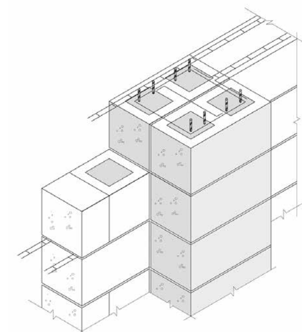
Figur 6.3 Vertikalarmert pilasterforsterking med Leca konstruksjonsblokk
