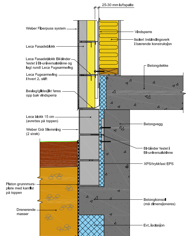
Figur 8.7 Forblending uten isolasjon. Vertikalt snitt
