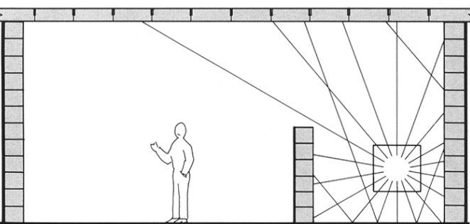
Figur 5.15 Skjematiske tegninger av lydstrålegang fra en støykilde i et lokale uten og med lydabsorberende Leca flater på tak, vegger og skjermer. Bare de to første refleksjonene er inntegnet. I det første tilfeller treffes mottakeren av et stort antall refleksjoner som gir et økt lydtrykknivå.
