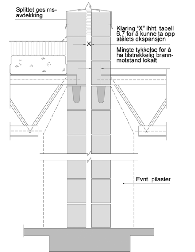
Figur 6.1 Lastbærende dobbel Leca seksjoneringsvegg
