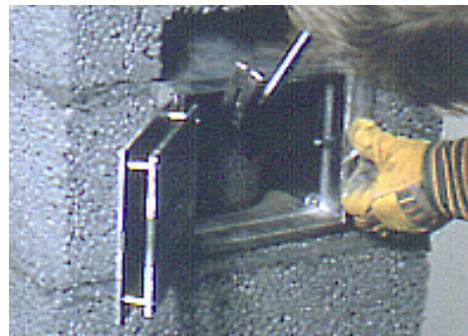
Bilde 4. Deretter festes feielukas karm med de to vedlagte stifter. Pass på at døra slår riktig vei før luka festes!
