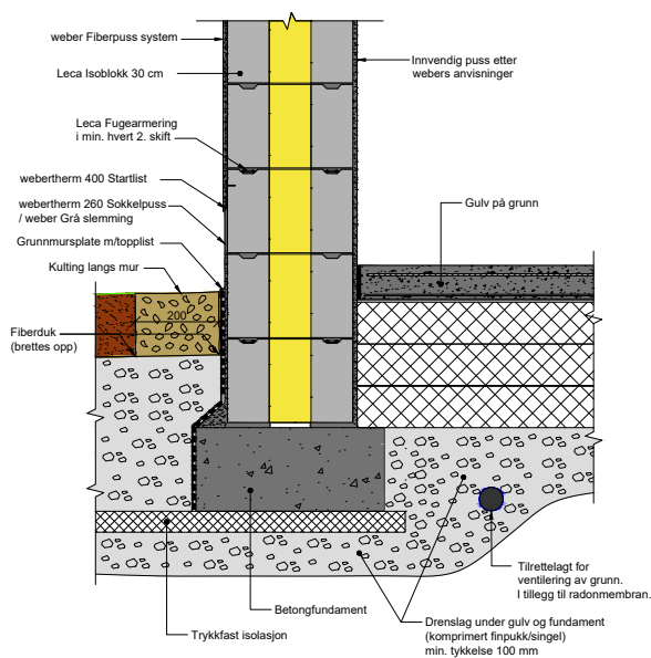
Figur 4.5 Veggopplegg på betongfundament
