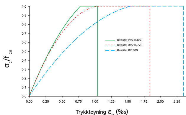
Figur 3.5 Karakteristisk arbeidsdiagram for Leca murverk med Leca Universalblokk ved vertikal trykkpåkjenning. Det antas at Leca LSX har tilsvarende verdier ved samme fasthet.
