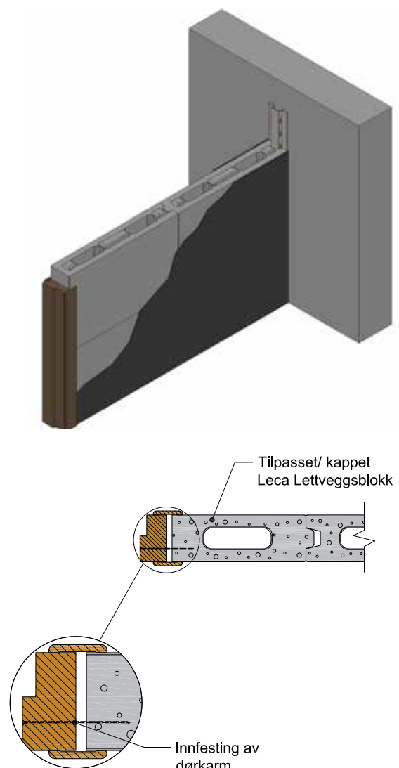
Figur 10.5d Innsetting av dør.
