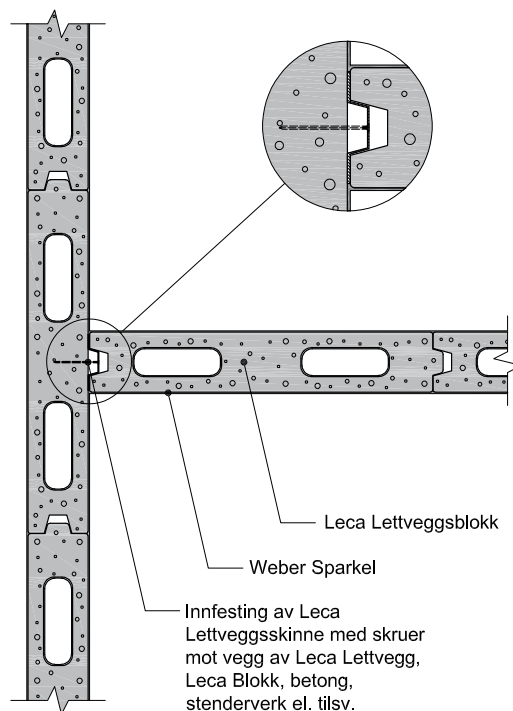
Fig. 10.3b Horisontalsnitt som viser innfesting av Leca Lettvegg mot en Leca Lettvegg ved bruk av Leca Lettveggsskinne og skruer/spiker. Skinnen blir dekket helt av sporet i Leca Lettveggsblokken.
