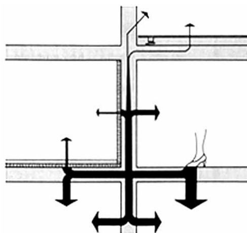
Figur 5.2 Trinnlydoverføring mellom rom i ferdig bygning
