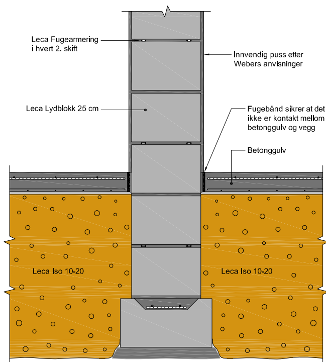
Figur 5.3 Betonggulv skilles fra lydskillevegg med fuger
