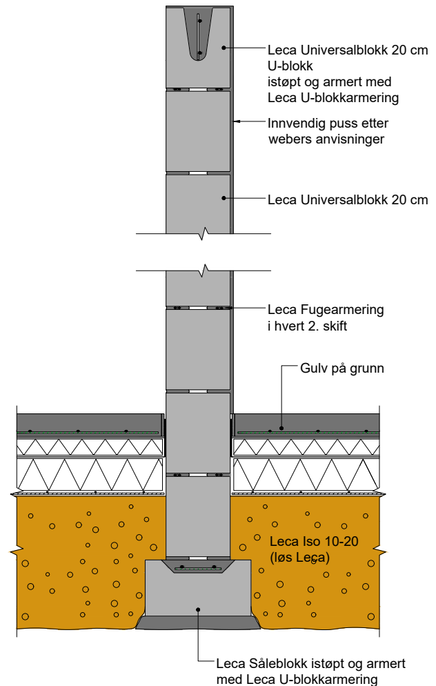
Figur 8.8 Innvendig bærevegg av Leca Universalblokk 20 cm. Vertikalt snitt.
