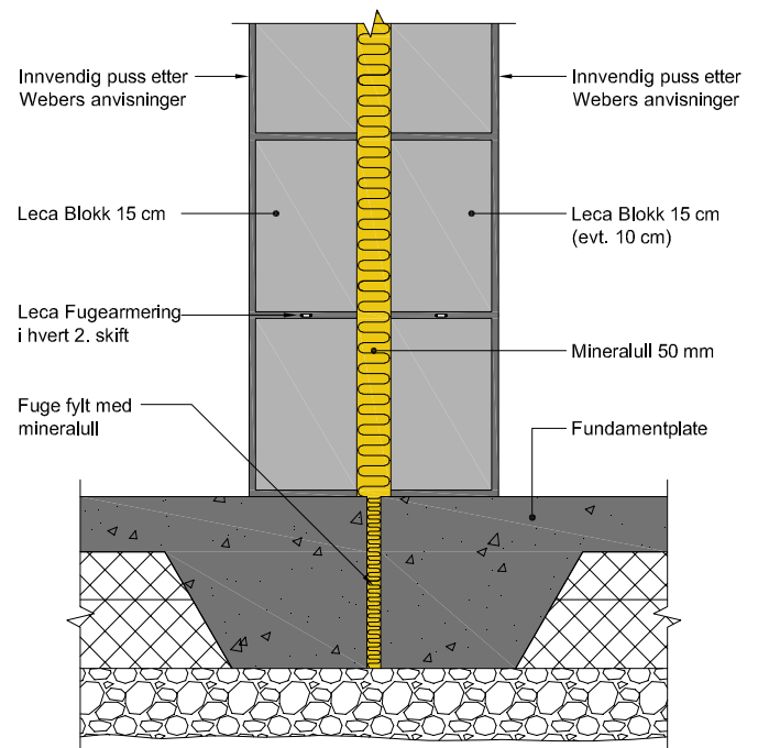
Figur 5.4 Dobbeltvegg av Leca Blokk 15 cm (10 cm)
