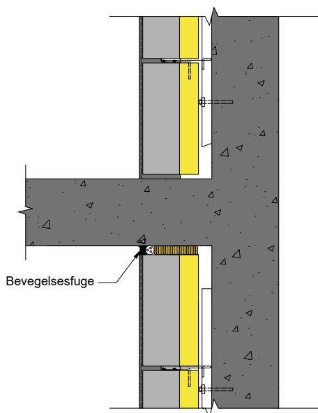
Figur 9.15 Fasadeblokk som møter utraget balkong eller takutstikk. NB! Det er ikke tatt hensyn til kuldebro.
