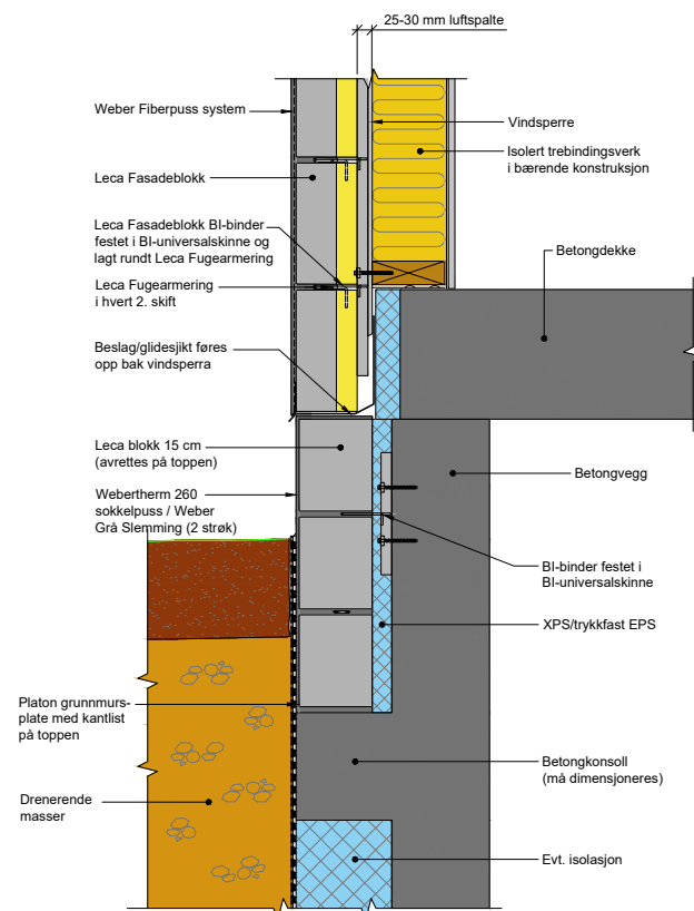
Figur 8.7 Forblending uten isolasjon. Vertikalt snitt.
