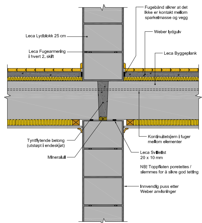
Figur 5.5 Endeskjøt over bærende lydskillevegg
