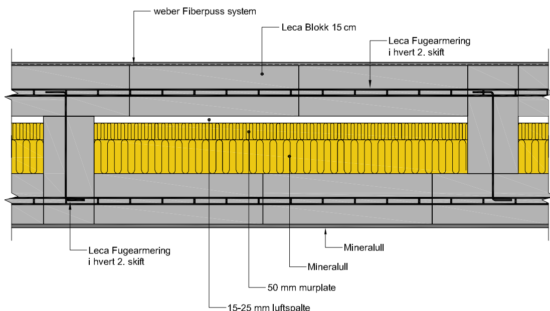
Figur 8.5 Diafragmavegg av Leca Blokk 15 cm. Plantegning
