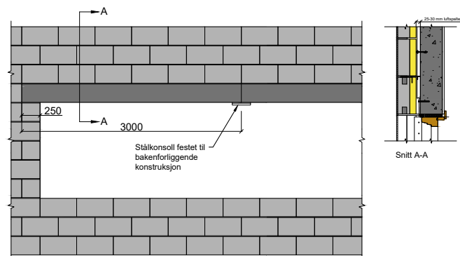
Figur 9.12 Prinsippskisse av overdekning som bæres av bygget
