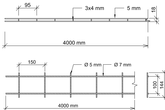
Figur 9.3a Leca Fugearmering og Leca U-blokkarmering
