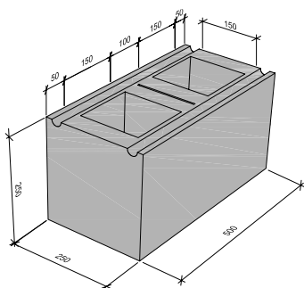
Figur 4.31 Leca Konstruksjonsblokk
