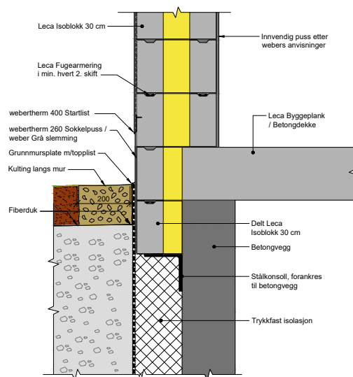
Figur 4.6 Leca murt på konsoll
