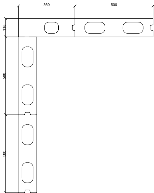
Figur 10.6a Første skift med Lettveggsblokk 118 mm. Forslag til kapping av hjørneblokk for å oppnå 1/2 blokks forband.
