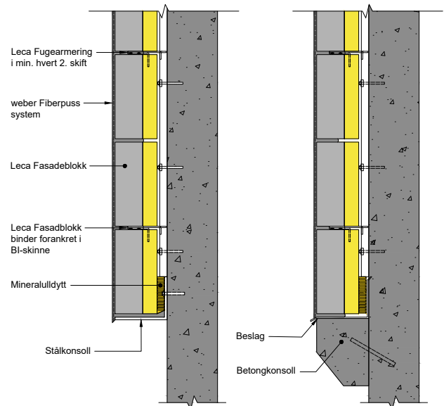
Figur 9.13 Utvendig forblending av «gammel» betongvegg. Opplegg på betong- og stålkonsoll.
