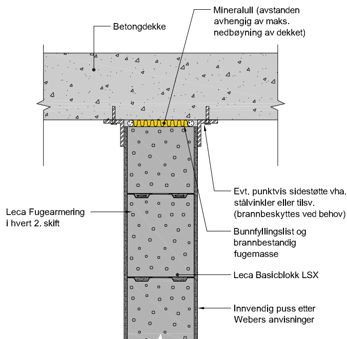
Figur 6.8 Leca brannseksjonerende vegg mot betongdekke
