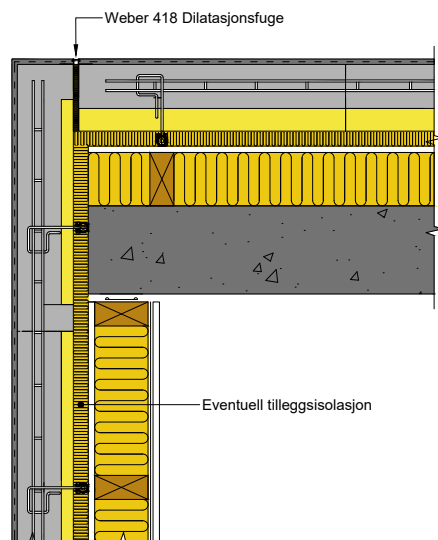
Figur 9.7 Forankring ved vertikal bevegesfuge i hjørne
