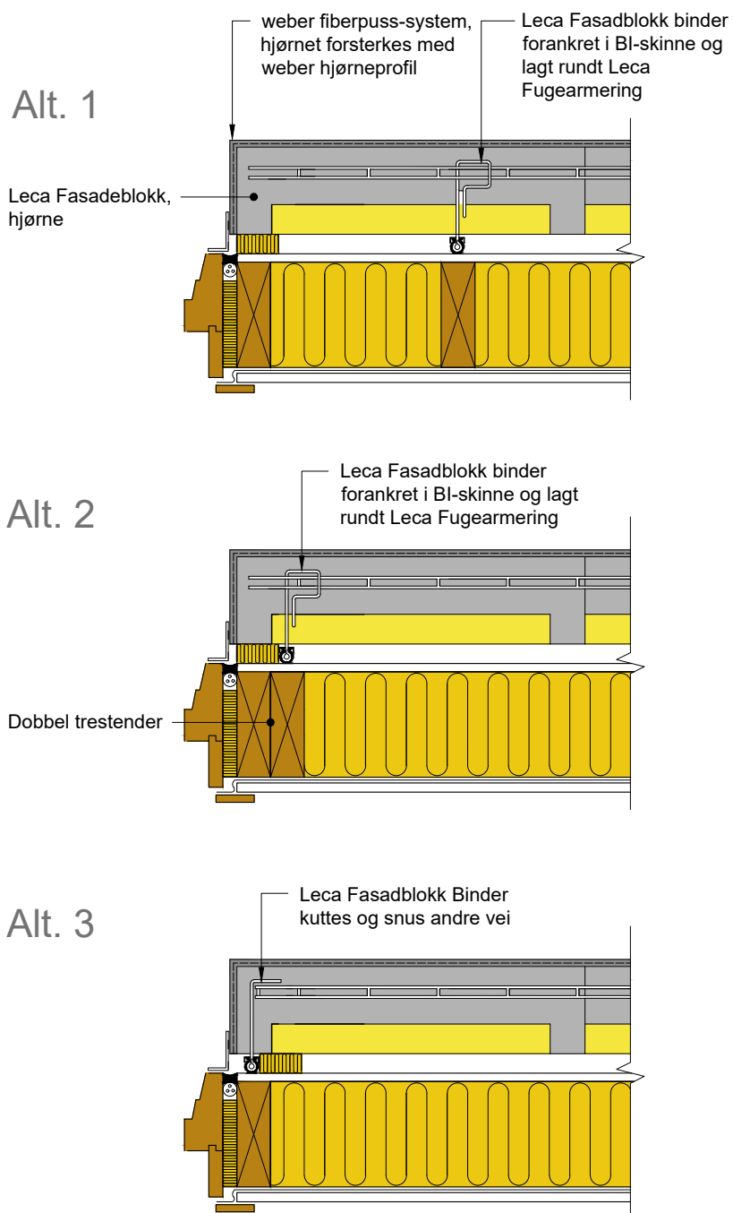
Figur 9.18 Vindusinnsetning i bakvegg av isolert bindingsverk – horisontalsnitt
