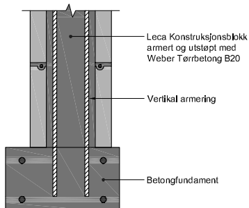
Figur 4.33a Vegg av Leca Konstruksjonsblokk. Fastholding i bunn og topp
