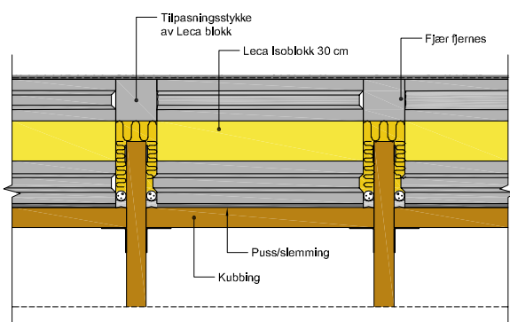
Snitt A-A (sett ovenfra)
