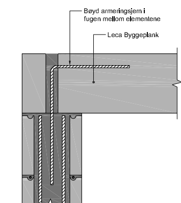
Figur 4.32 Murverk av Leca Konstruksjonsblokk. Armert og utstøpt
