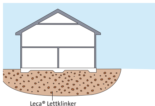
Fig. 5.4.1: Kompensert fundamentering med Leca® Lettklinker.
