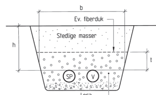
Figur 9.4: Leca®ISO 8/20 er brukt i hele omfyllingen.
