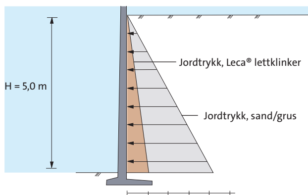
Fig. 6.6.2: Støttemur med Leca® Lettklinker som lett tilbakefylling
