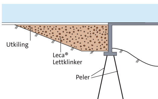
Fig. 5.2.2: Leca® Lettklinker som tilbakefylling mot brulandkar gir belastningsreduksjon på underliggende naturlige masser og hindrer setningsdifferanser.
