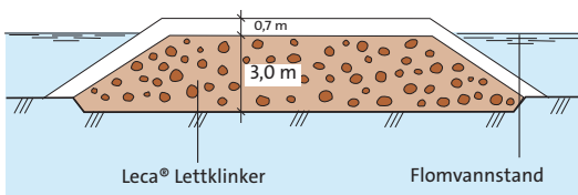
Fig. 6.3 Veifylling som blir utsatt for flom like etter utlegging.
