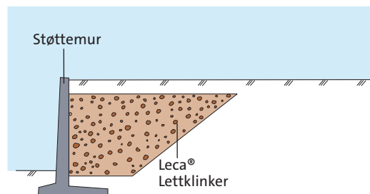
Fig. 5.3.1: Støttemur med Leca® Lettklinker som lett tilbakefylling
