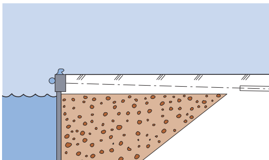
Fig. 10.1.1: Typisk snitt gjennom en spuntveggs kai hvor det er benyttet Leca® Lettklinker som lett fyllmasse.
