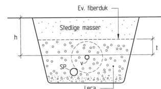
Figur 9.5: For mindre sekundær- og stikkledninger kan det være nødvendig å isolere vannledningen fra grøttebunnen.
