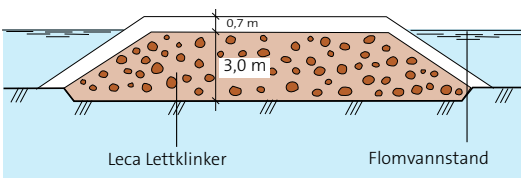
Fig. 6.3 Veifylling som blir utsatt for flom like etter utlegging.
